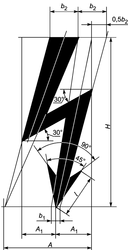
Рисунок Н.1 - Графический символ электрического напряжения
