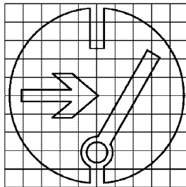
Рисунок П.3 - Предписывающие знаки
